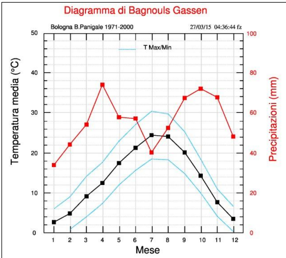
Figura 5-1: Diagramma ombrotermico (Bagnouls e Gausson, 1957, Walter e Lieth, 1960-67) relativo alla stazione di Bologna B. Panigale
