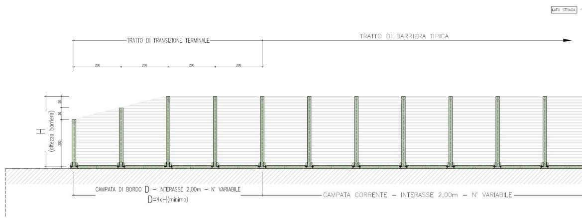
Figura 3-5. Transizione terminale H= 3m – Lato strada
