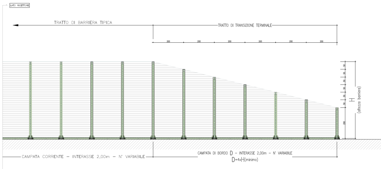
Figura 3-10. Transizione terminale H= 5m – Lato ricettore
