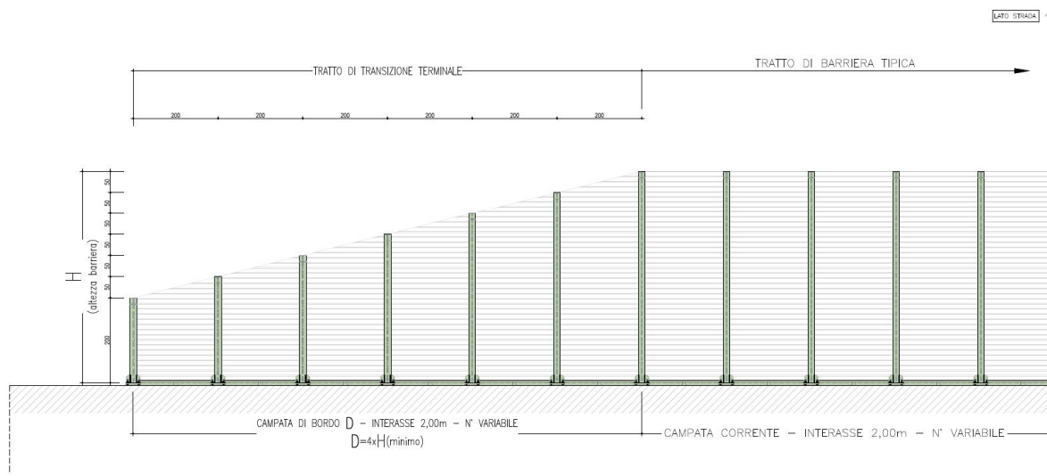
Figura 3-9. Transizione terminale H= 5m – Lato strada
