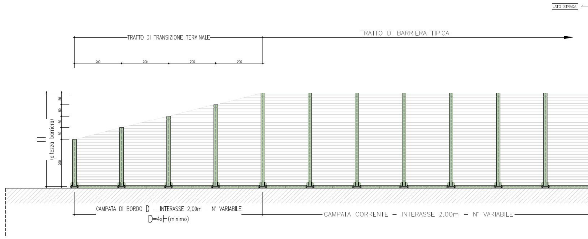
Figura 3-7. Transizione terminale H= 4m – Lato strada
