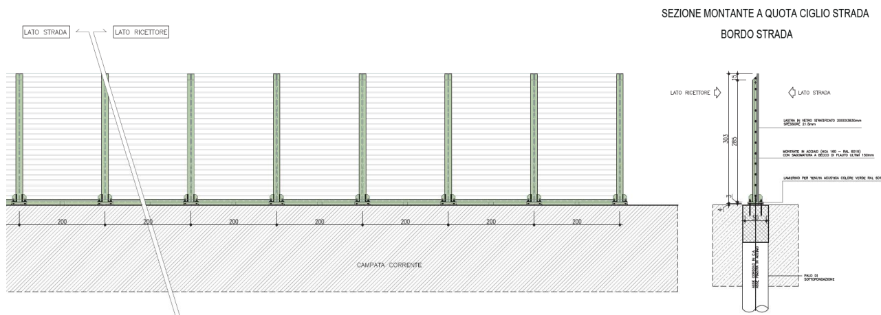
Figura 3-11. Barriera Tipo 1A - Trasparente H=3m
