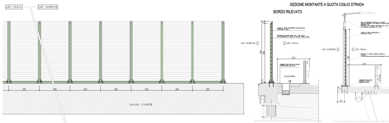
Figura 3-12. Barriera Tipo 1B - Trasparente H=4m
