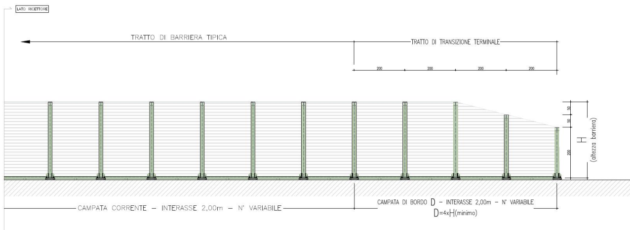
Figura 3-6. Transizione terminale H= 4m – Lato ricettore
