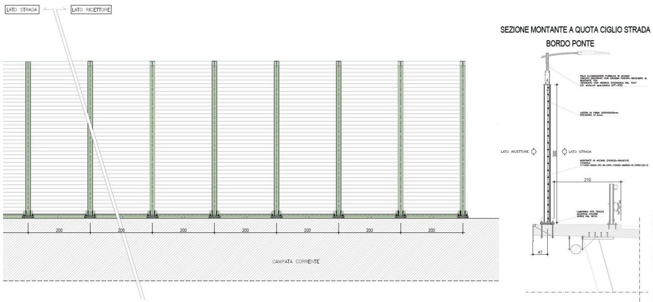
Figura 3-13. Barriera Tipo 1C - Trasparente H=5m
