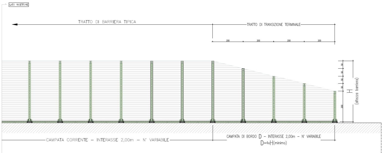
Figura 3-8. Transizione terminale H= 4m – Lato ricettore
