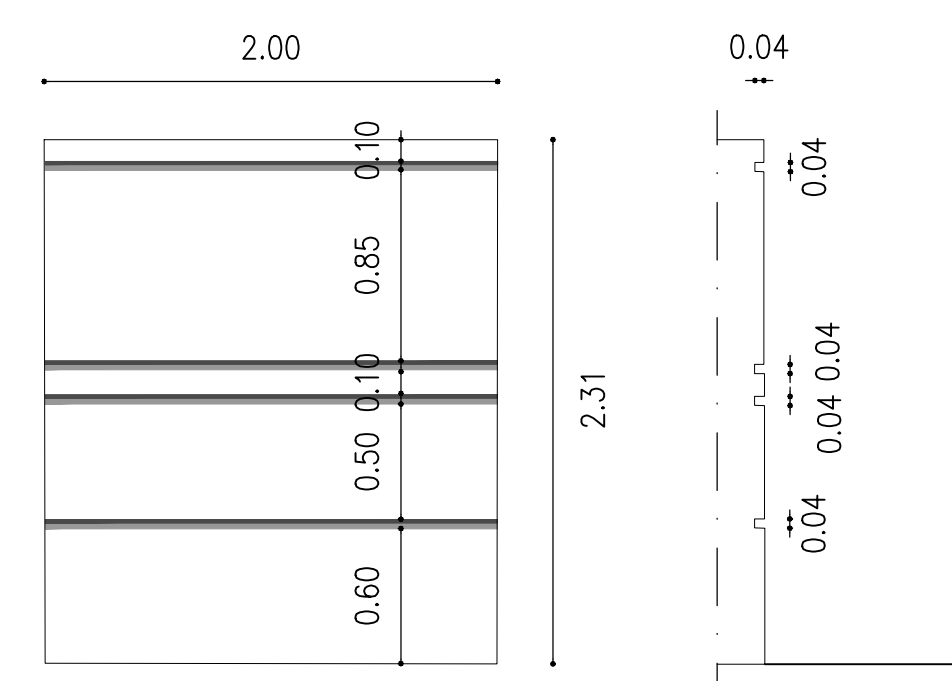
NOTA SU DETTAGLIO ARCHITETTONICO MURI
