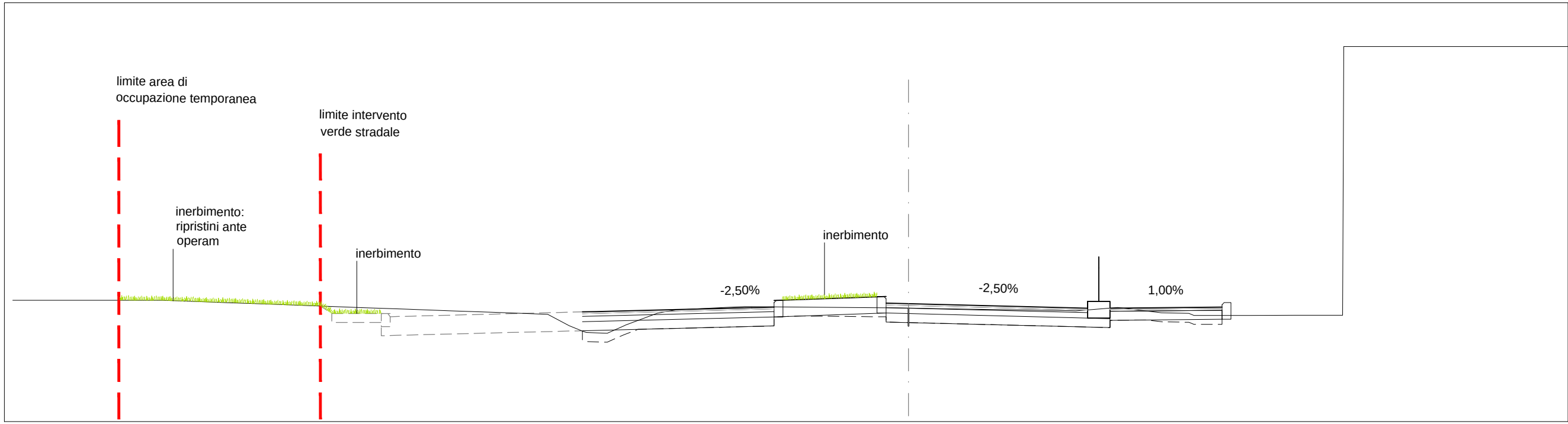
Sezione 9 Tratto RP01 - scala 1:100
