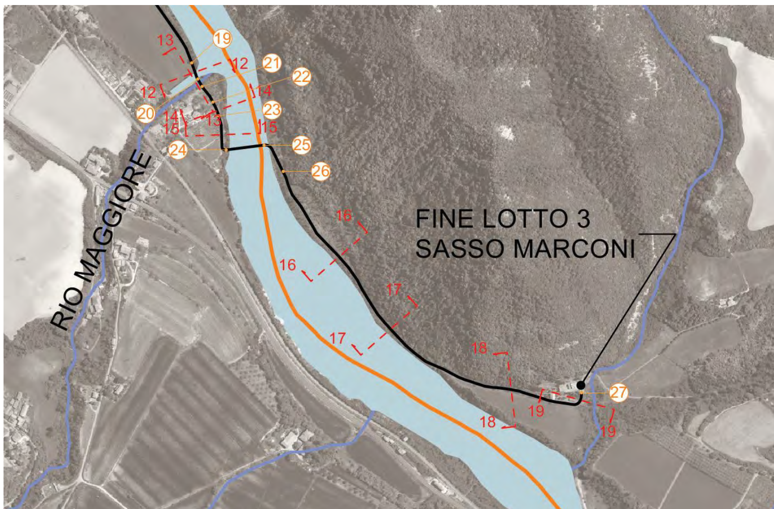
FIGURA 2.4.2.1 - ILLUSTRAZIONE DELLA POSIZIONE DELLE SEZIONI LUNGO IL TRACCIATO DELLA CICLOVIA.
