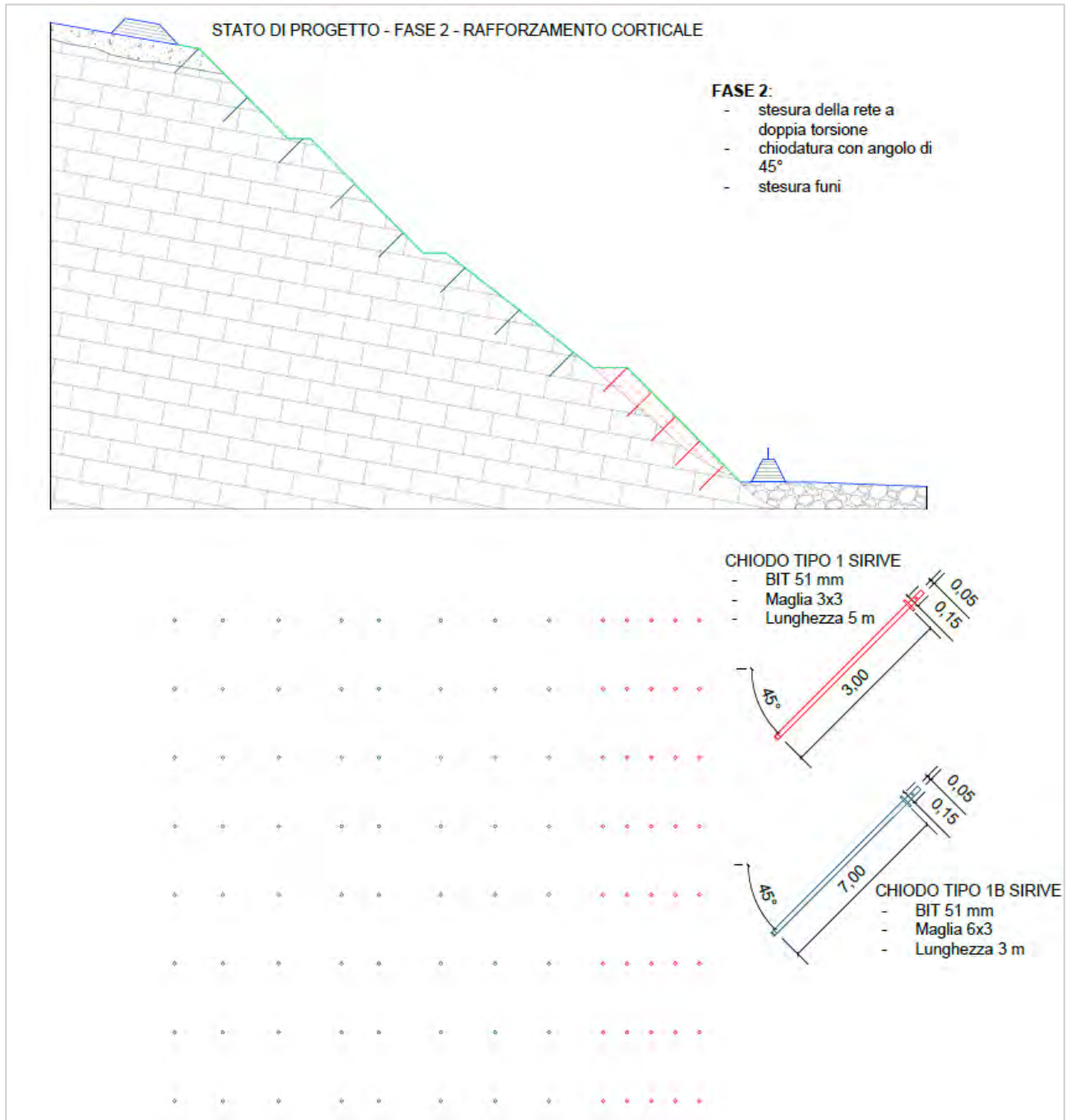
FIGURA 2.4.4.4 - FASE 2 DI MESSA IN SICUREZZA VERSANTE.
