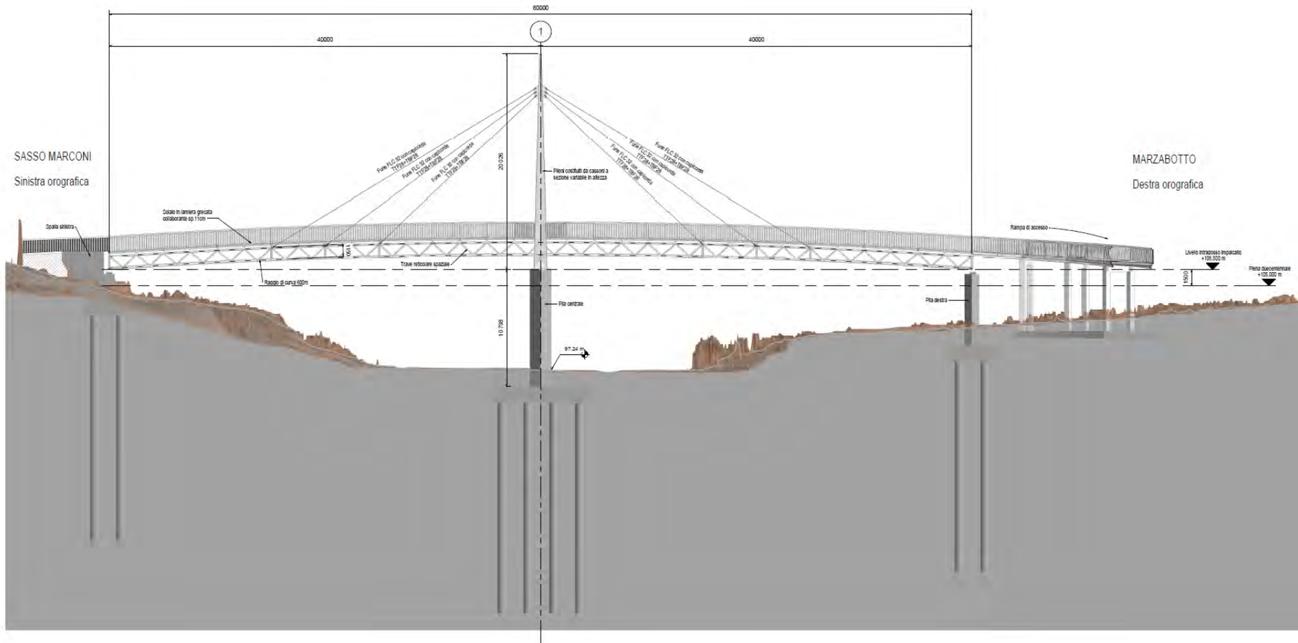
FIGURA 2.4.3.3 - PROSPETTO LONGITUDINALE DELLA PASSERELLA SUL RENO
