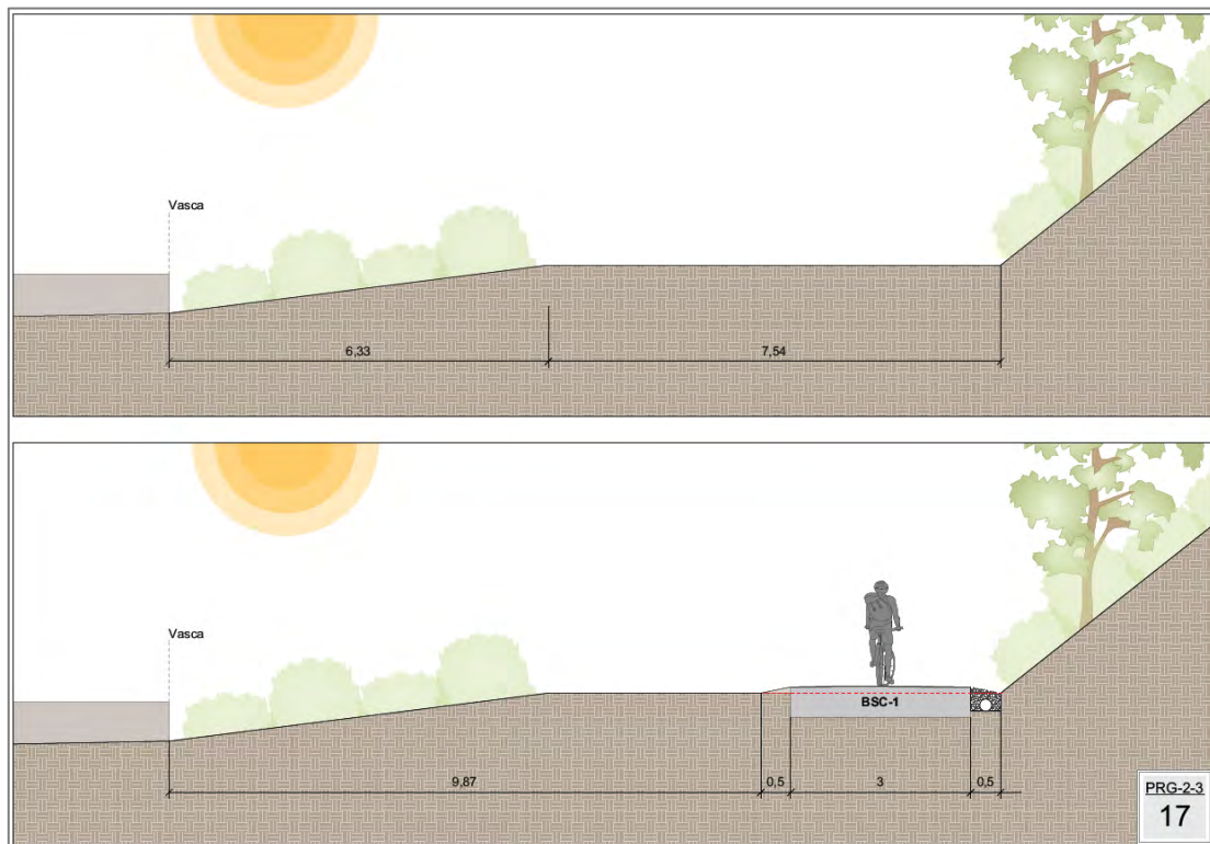
FIGURA 2.4.2.3 - SEZIONE 17.
