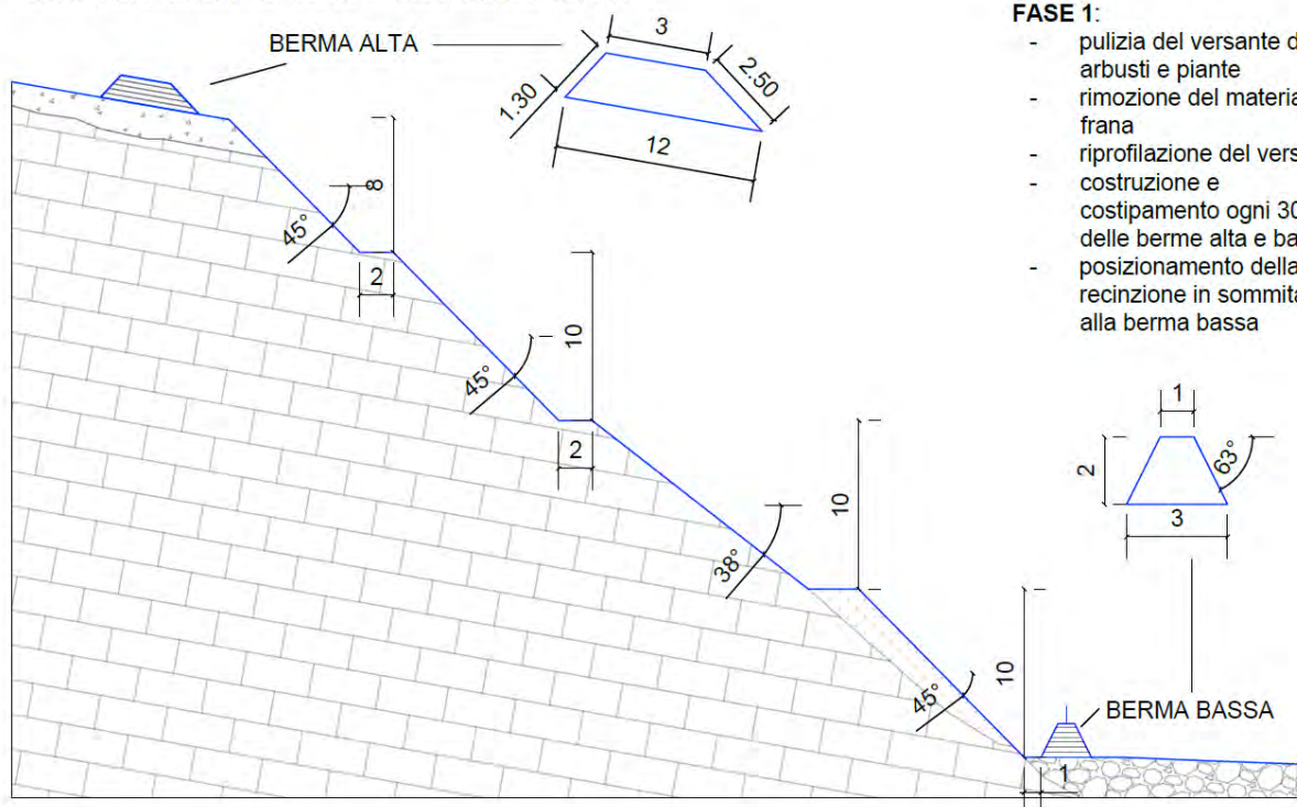
FIGURA 2.4.4.3 - FASE 1 DI MESSA IN SICUREZZA VERSANTE.
