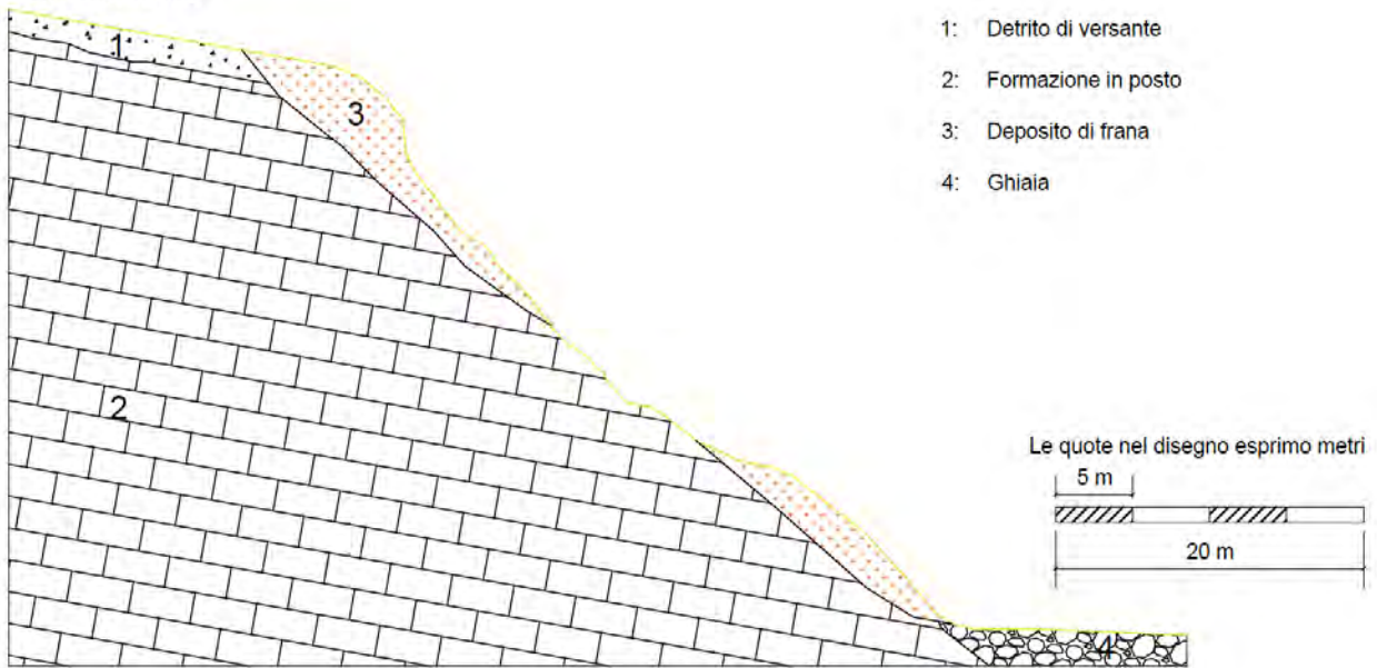
FIGURA 2.4.4.2 - STATO DI FATTO FRANA.
