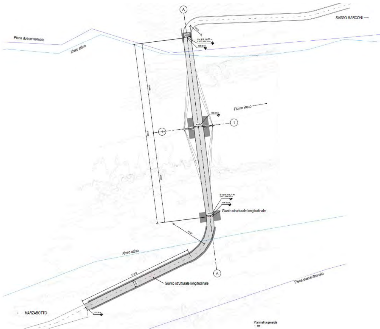
FIGURA 2.4.3.1 - PLANIMETRIA GENERALE DELLA PASSERELLACICLOPEDONALE SUL FIUME RENO.
