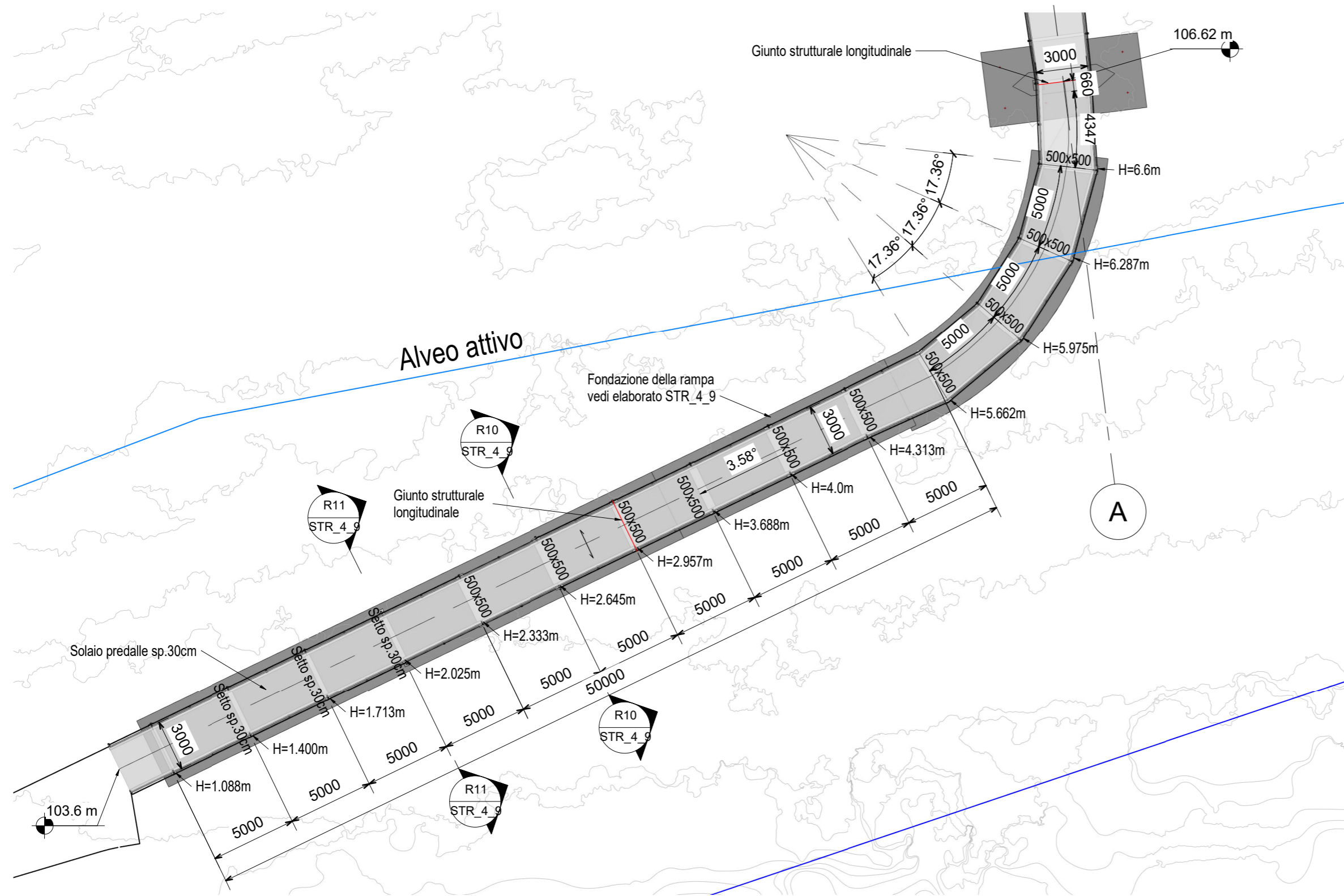
Pianta - Rampa Sud 1 : 250
