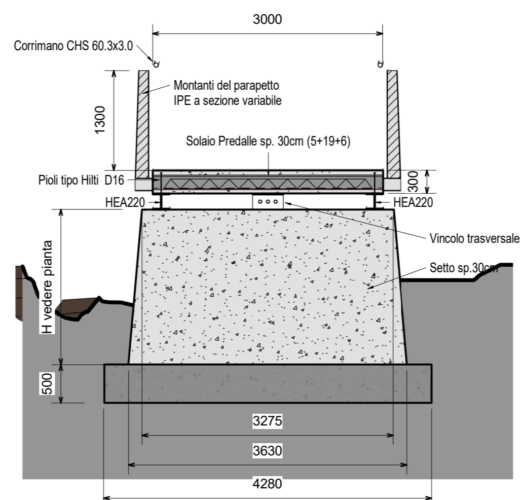
Sezione R11 - Sezione tipica a setto 1 : 50
