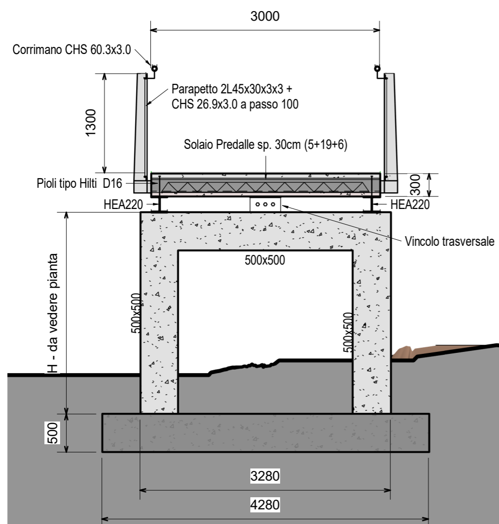
Sezione R10 - Sezione tipica a telaio 1 : 50
