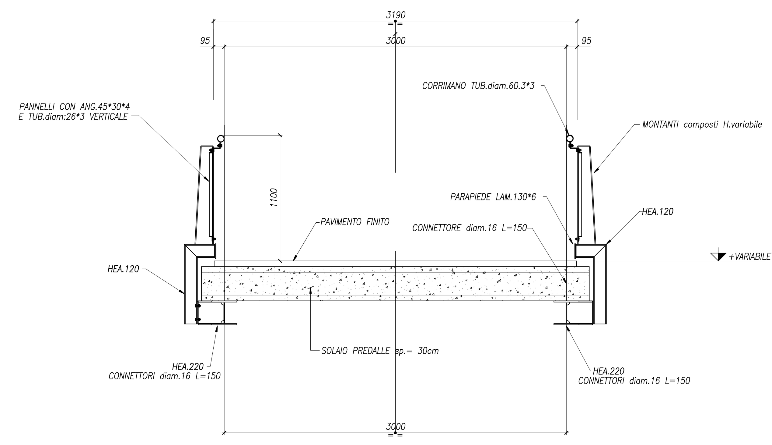
SEZIONE TRASVERSALE E-E
