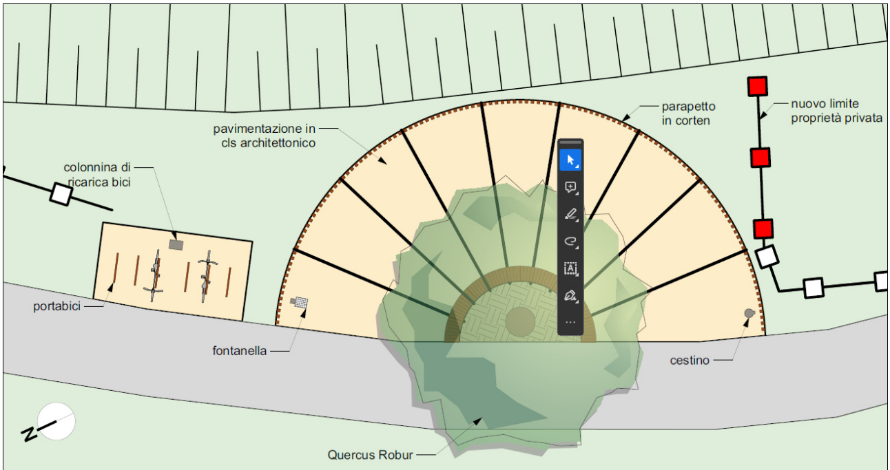
Figura 22. Planimetria di progetto dell’area di sosta laghetti di Porziola (elaborato INT-1-1)
