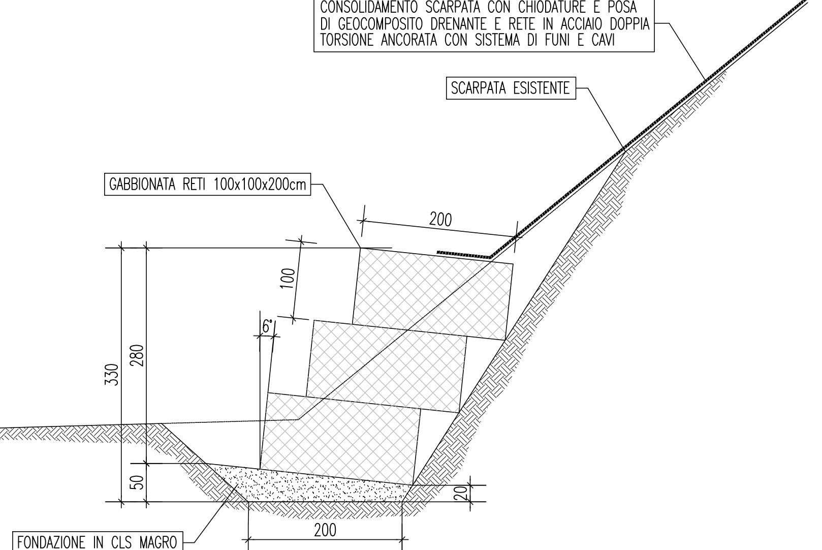
GABBIONATA A VALLE SEZIONE TIPO Scala 1:50
