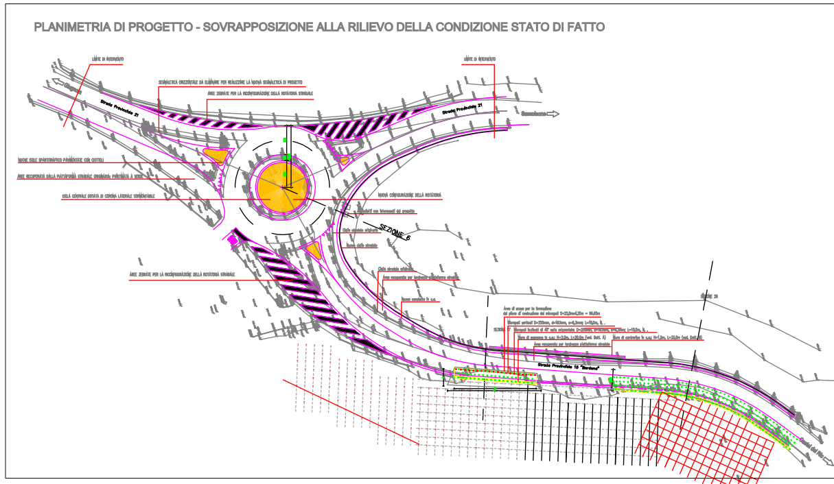
Figura 19: planimetria di progetto sovrapposta al rilievo topografico della strada dal km0+00 al franco.
