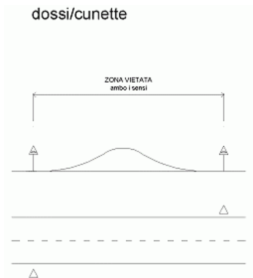
Figura 4. Art. 5 comma 2 del Regolamento: Raccordi verticali concavi e convessi segnalati
