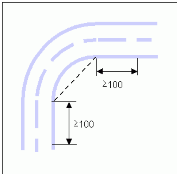
Figura 7. Art. 5 comma 3 del Regolamento: Curva e relative distanze
