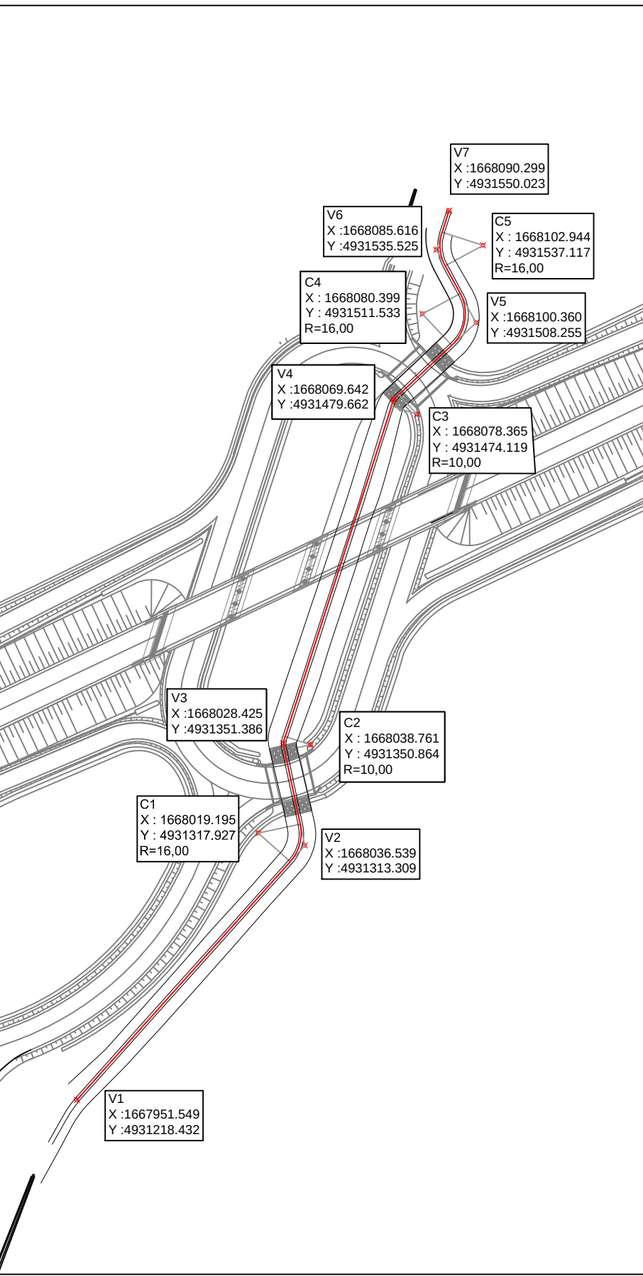
Planimetria di tracciamento Scala 1:2.000
