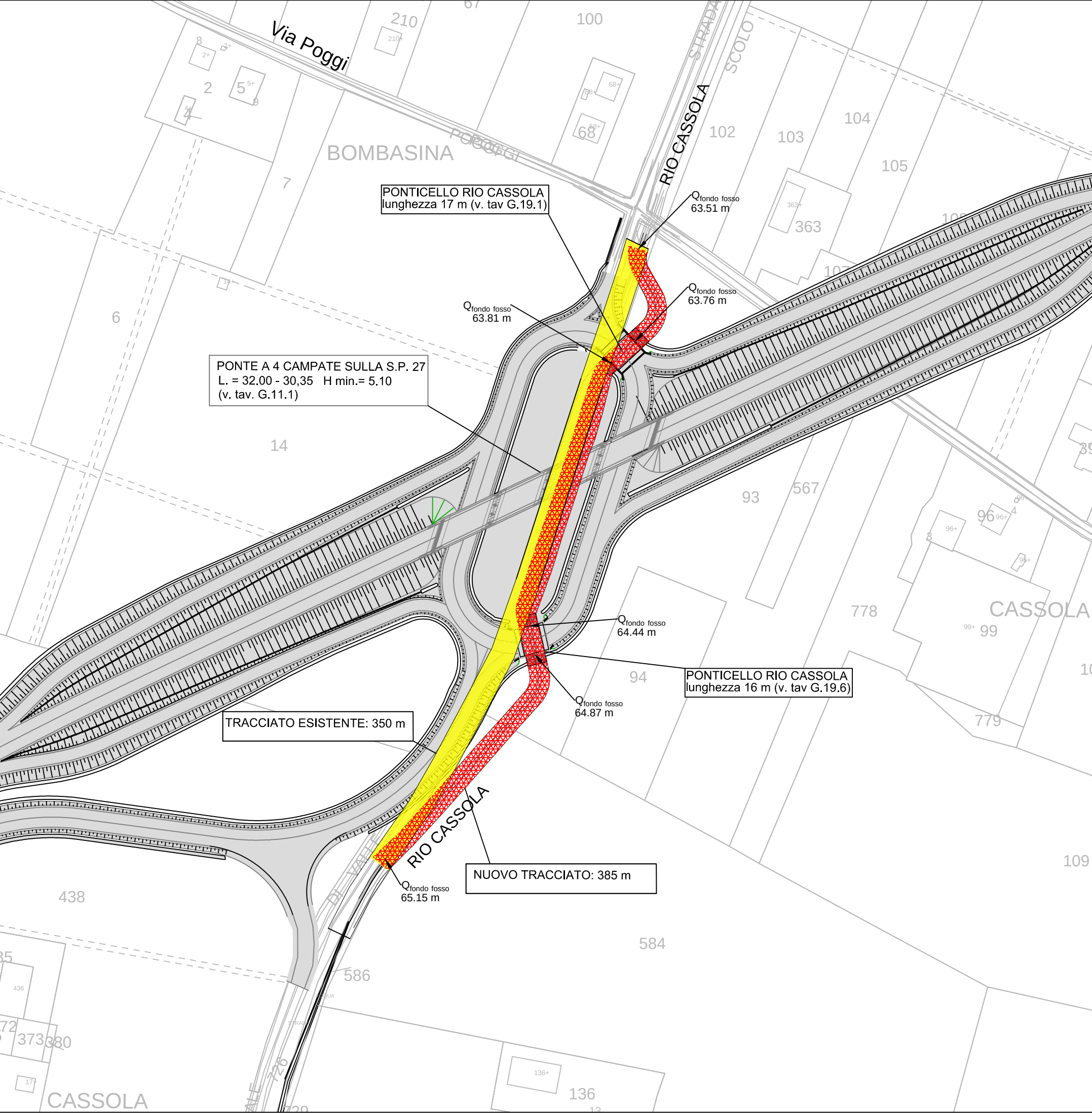
Planimetria catastale Scala 1:1.000
