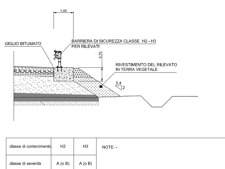
barriera metallica su cordolo (H70xL100) SCALA 1:100
