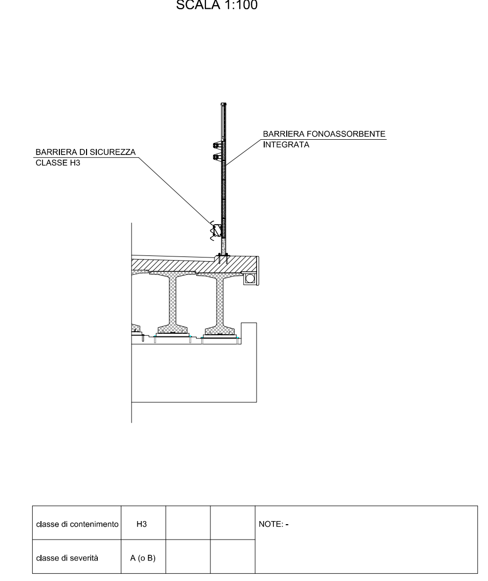
barriera metallica con barriera acustica combinata SCALA 1:100
