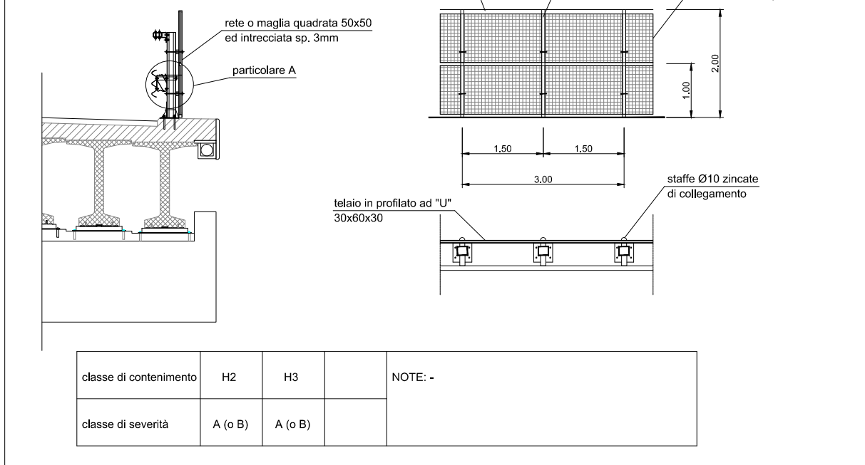
barriera metallica con rete metallica parasassi SCALA 1:100
