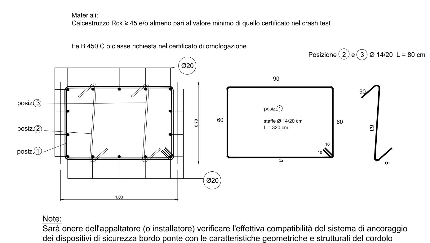
PARTICOLARE B - Cordolo di fondazione 70 x 100 FUORI SCALA
