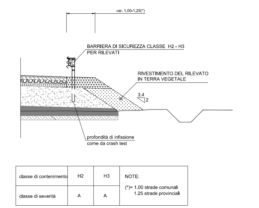
barriera metallica su scarpata con pendenza 2/3,4 e altezza > 2.00 SCALA 1:100
