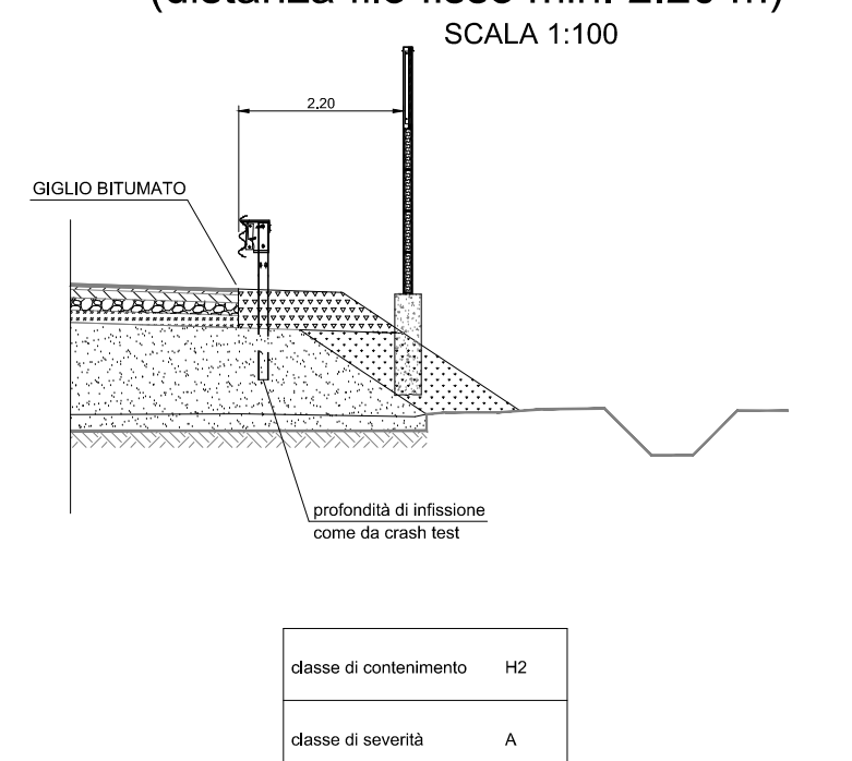
barriera metallica con barriera acustica a tergo (distanza filo fisso min. 2.20 m) SCALA 1:100
