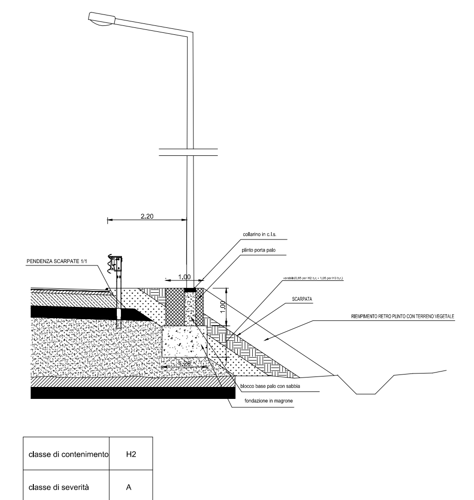
barriera metallica con palo di illuminazione a tergo SCALA 1:100
