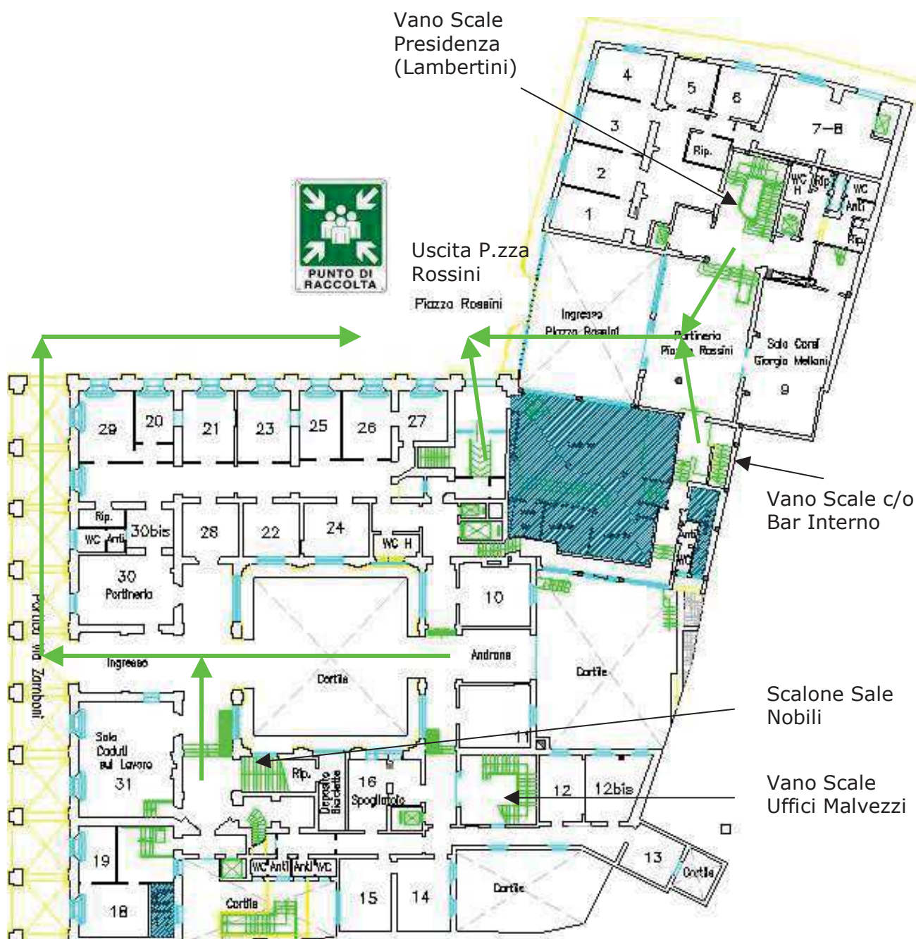
Pianta del piano terra, localizzazione del punto di raccolta e delle principali vie d'esodo. Nelle Bacheche sono affisse le piante di evacuazione con l'indicazione di TUTTI i percorsi mentre qui sono indicate solo le vie principali
