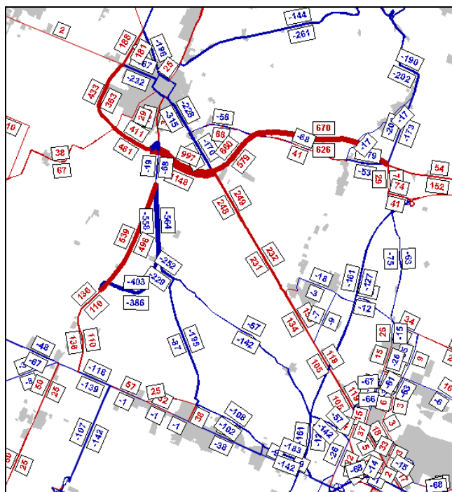
Figura 58: Configurazione infrastrutturale PERSICETANA - Rete di differenza
