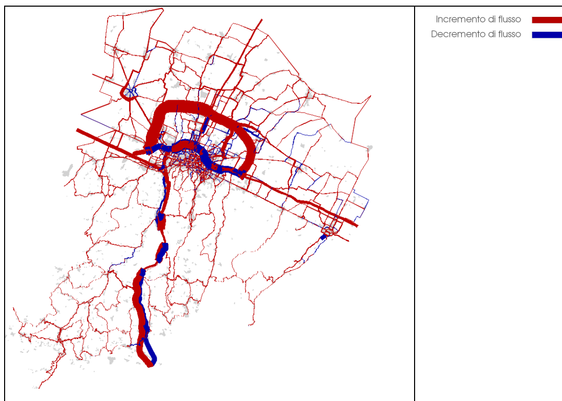
Figura 5: Variazioni di flussi tra lo Scenario di riferimento e lo Stato attuale
