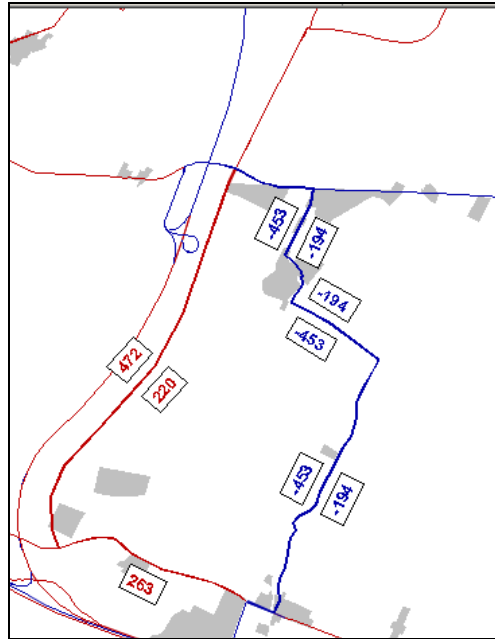
Figura 81: Configurazione infrastrutturale ZENZALINO - Rete differenza con intervento 10a
