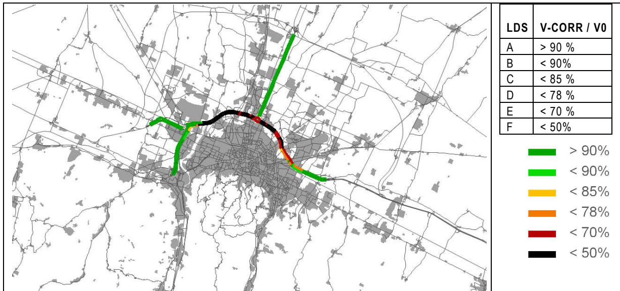
Figura 31: Scenario di riferimento - Livello di Servizio del sistema tangenziale
