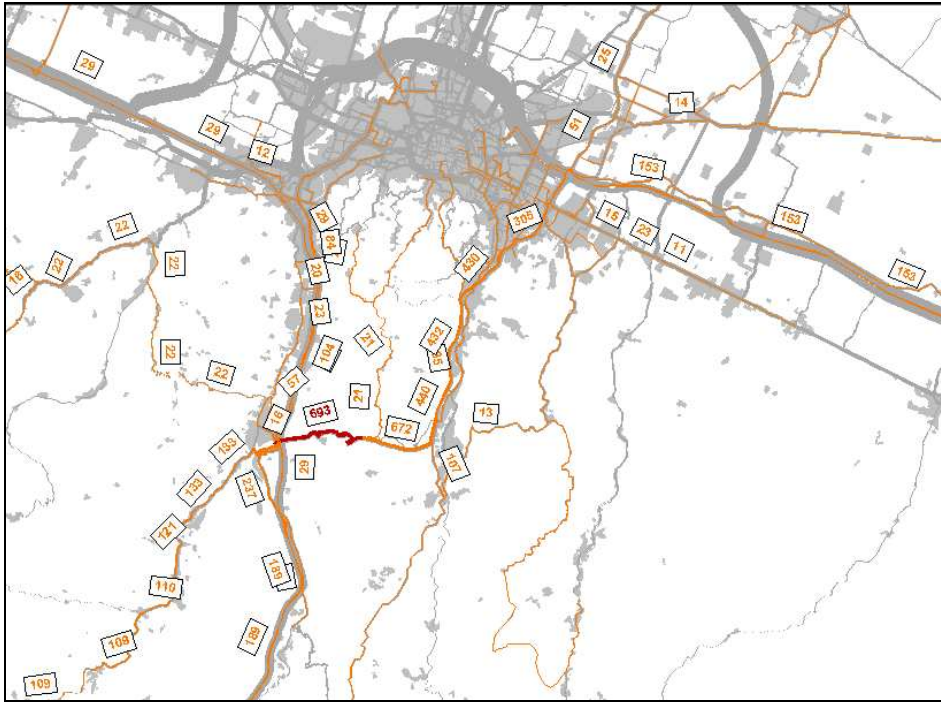
Figura 77: Composizione infrastrutturale SAVENA - Composizione di flusso su SP37 dir. Ovest-Est
