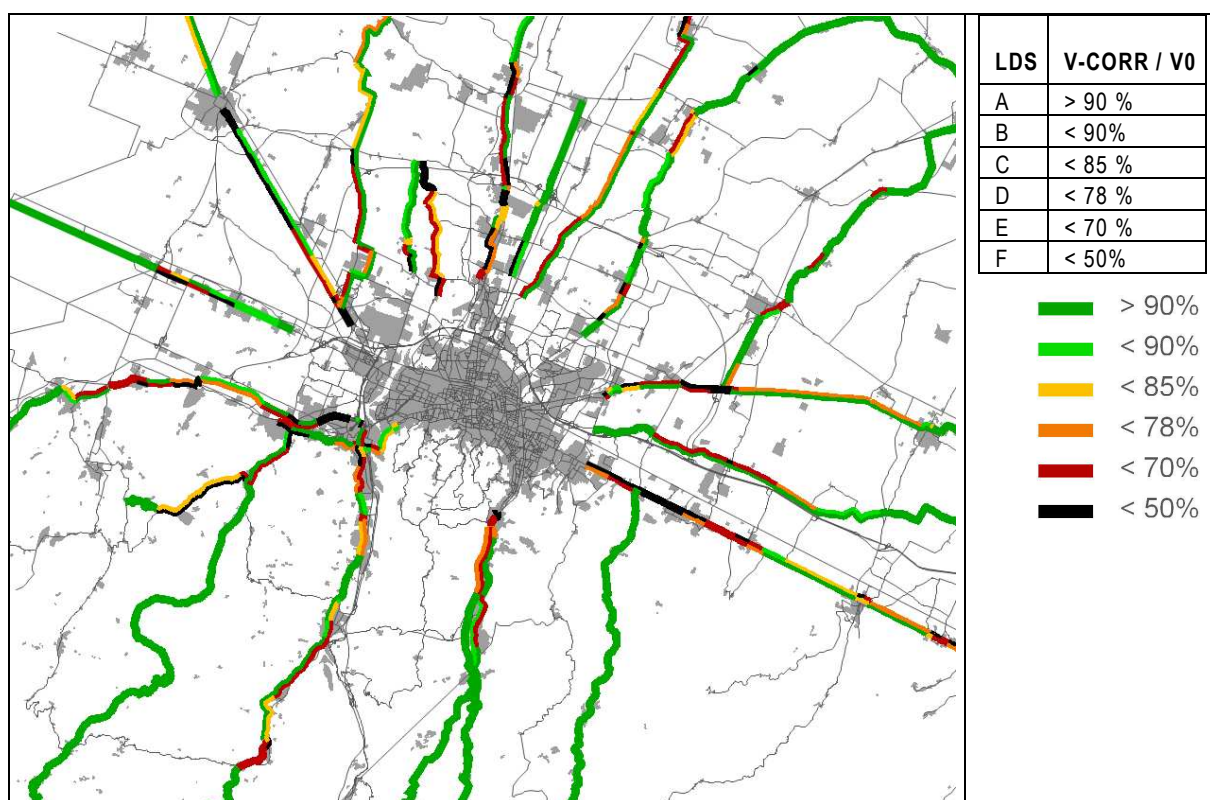
Figura 36: Scenario di riferimento - Livello di Servizio delle principali radiali
