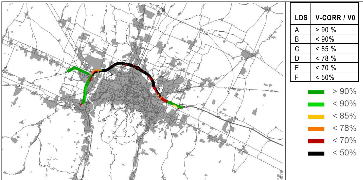
Figura 14: Stato attuale: Livello di Servizio del sistema tangenziale
