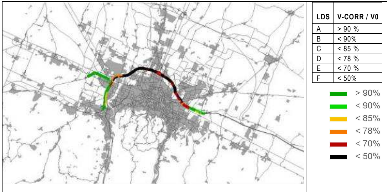
Figura 30: Scenario tendenziale - Livello di Servizio del sistema tangenziale
