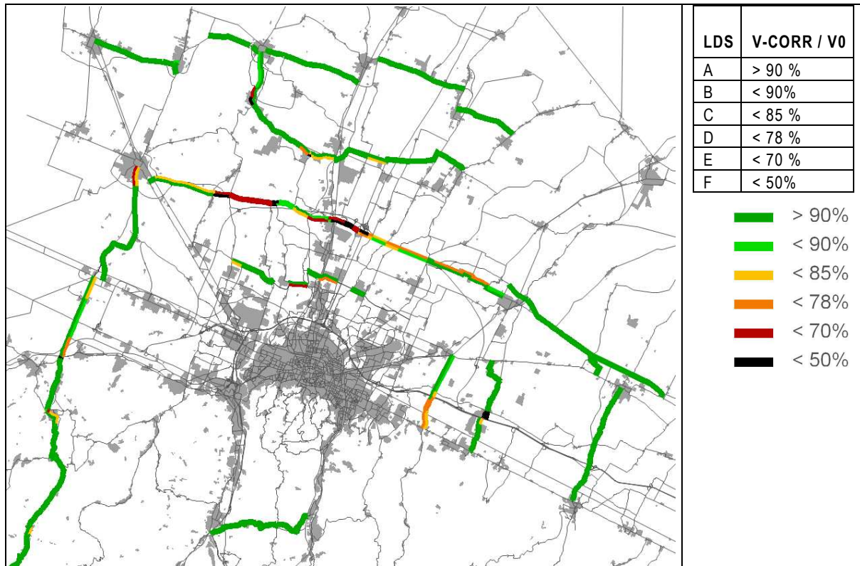
Figura 16: Stato Attuale: Livello di Servizio delle principali trasversali
