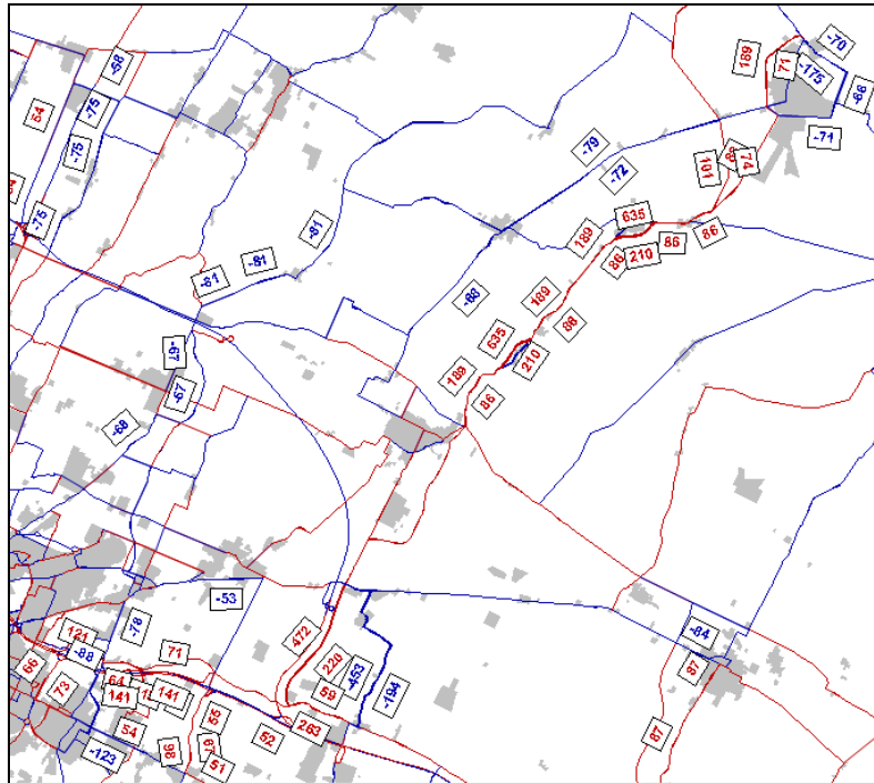
Figura 80: Configurazione infrastrutturale ZENZALINO - Rete di differenza
