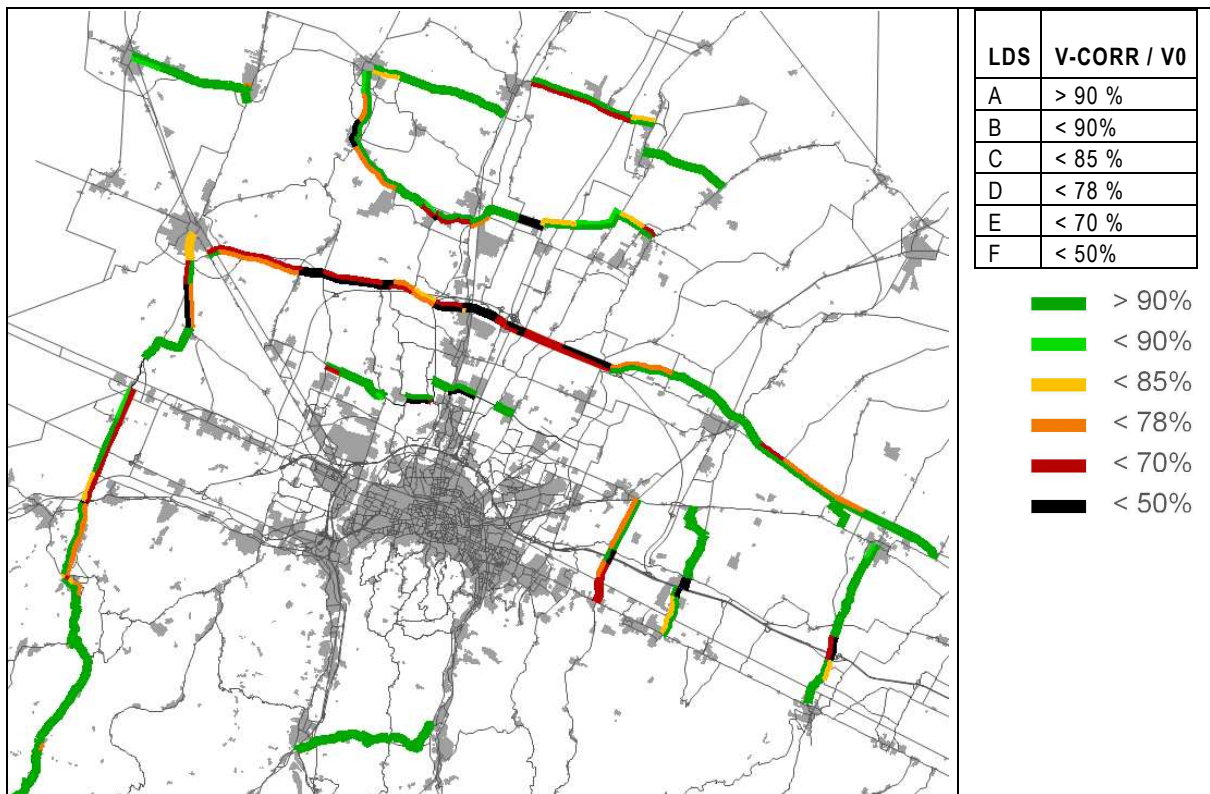
Figura 37: Scenario tendenziale - Livello di Servizio delle principali trasversali
