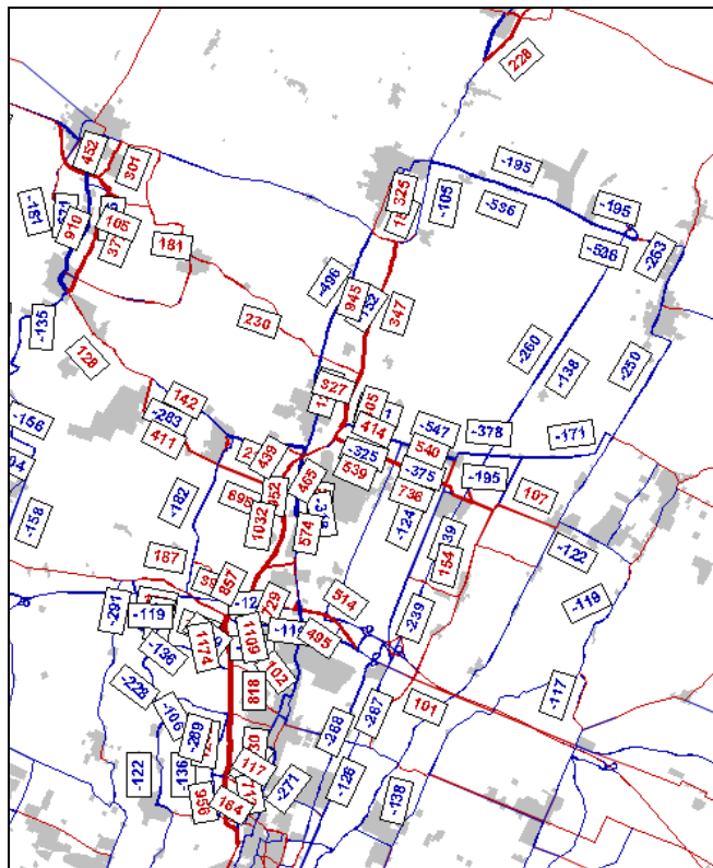
Figura 68: Configurazione infrastrutturale NUOVA GALLIERA - Rete di differenza
