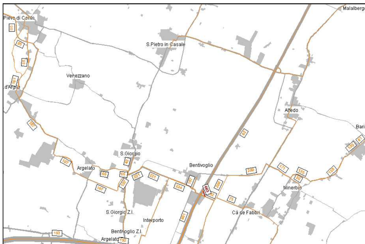
Figura 86: Configurazione infrastrutturale BASSA BOLOGNESE - Composizione di flusso sul casello di Bentivoglio (ingresso)
