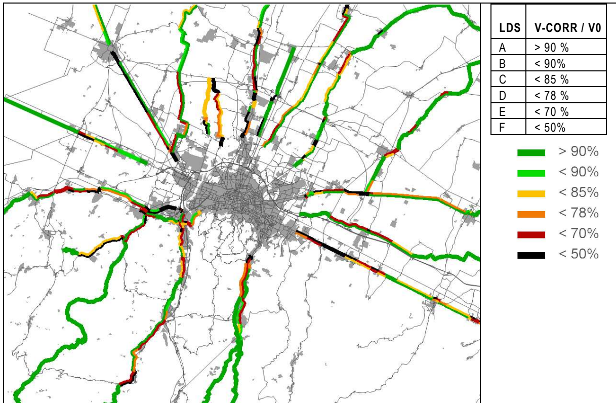
Figura 35: Scenario tendenziale - Livello di Servizio delle principali radiali
