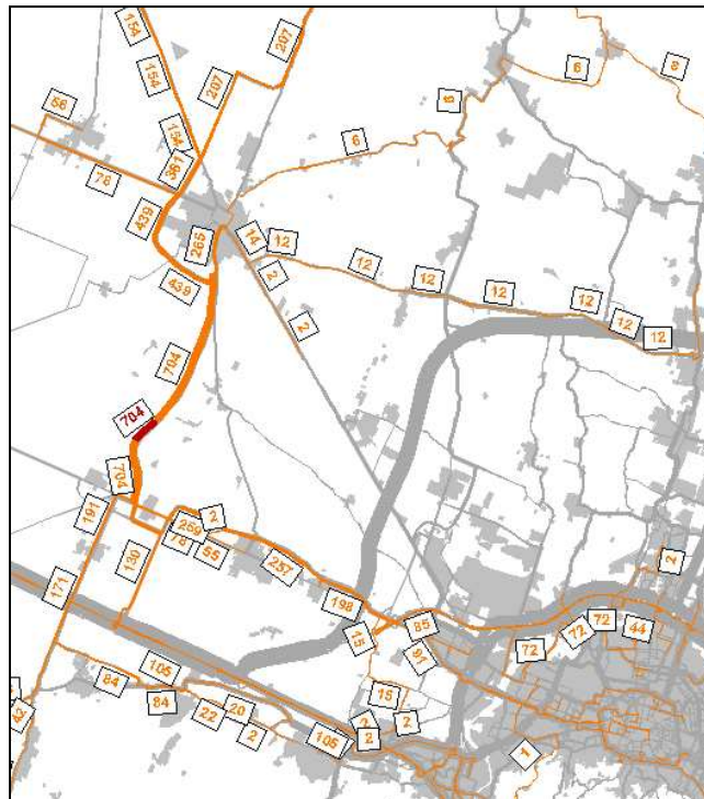
Figura 57: Corridoio EMILIA PONENTE - Composizione di flusso lungo la SP2 dir. Nord-Sud
