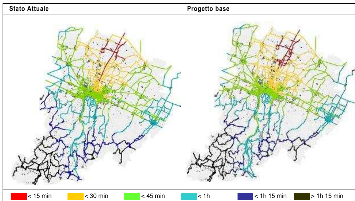
Figura 108: Accessibilità al sistema autostradale – portale A13
