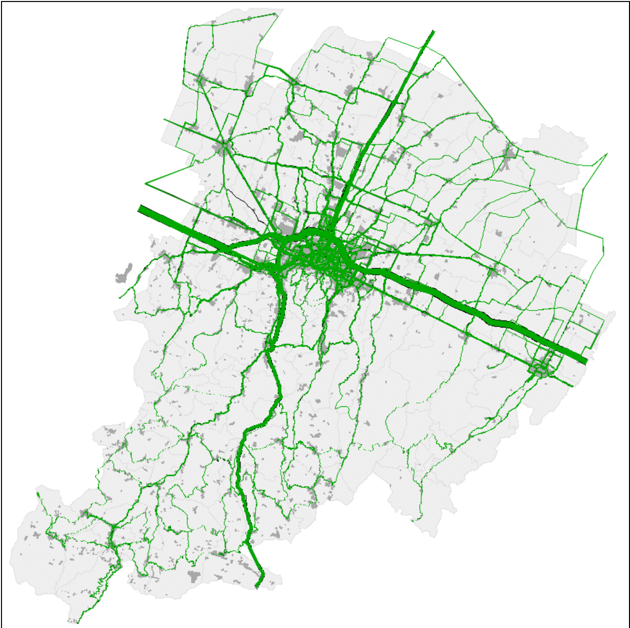
Figura 8: Flussogramma veicoli leggeri 08:00 – 09:00
