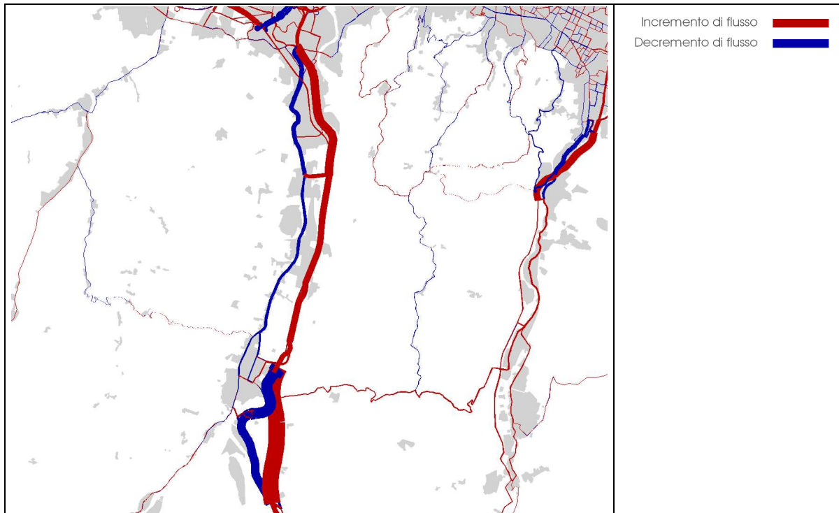
Figura 101: Nuova Porrettana: variazioni di flussi fra lo scenario di progetto base e lo scenario attuale
