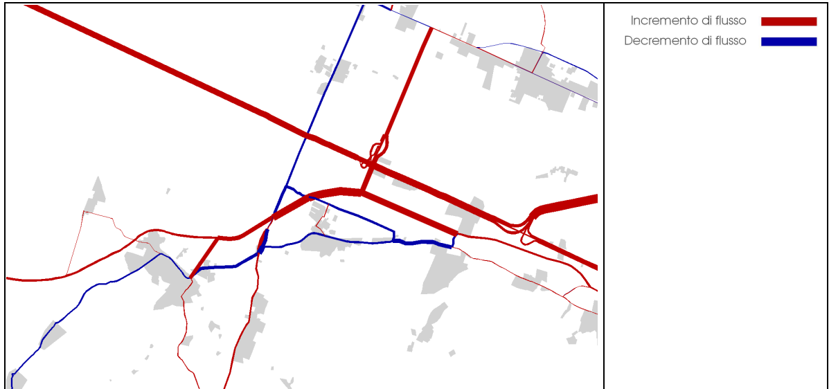
Figura 102: Nuova Bazzanese - variazioni di flussi fra lo scenario di progetto base e lo scenario attuale
