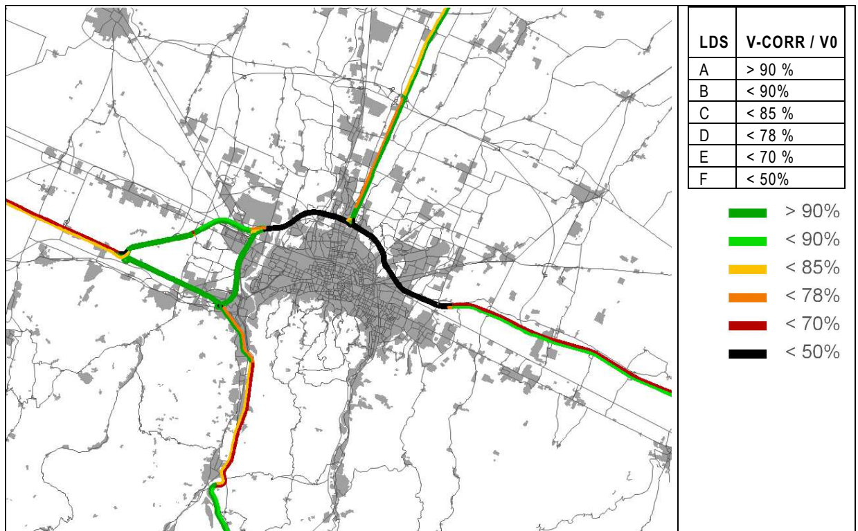
Figura 13: Stato attuale: Livello di Servizio del sistema autostradale
