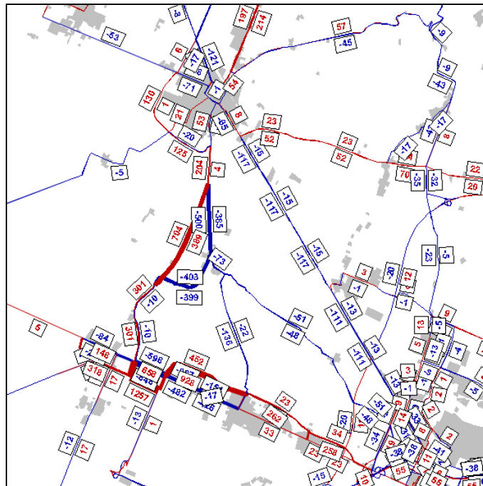
Figura 56: Configurazione infrastrutturale EMILIA PONENTE - Rete di differenza
