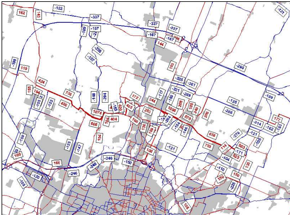
Figura 62: Configurazione infrastrutturale INTERMEDIA DI PIANURA - Rete di differenza (valori > 100)
