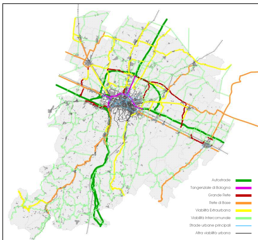
Figura 2: Scenario di riferimento - Assetto funzionale della rete viaria
