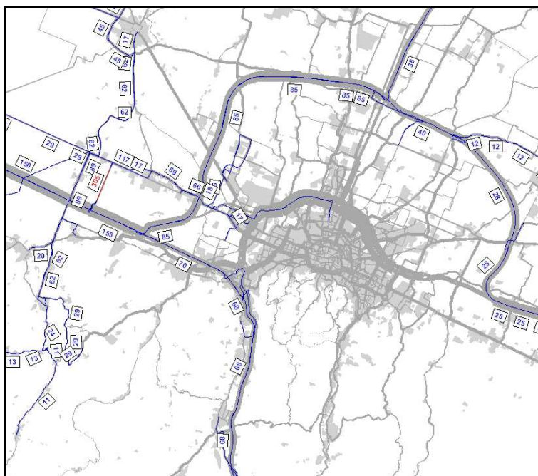
Figura 14: Collegamento via Emilia-casello della Muffa - Composizione di flusso da casello della Muffa a via Emilia
