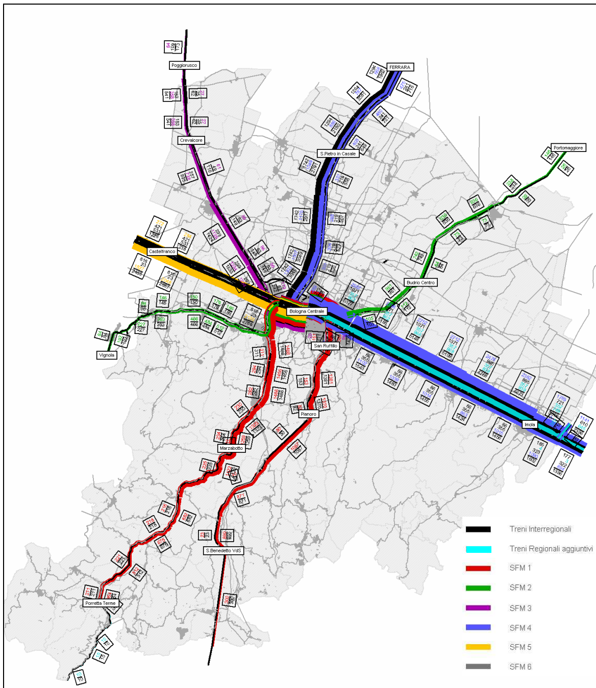
Figura 25: Scenario di Riferimento - Flussogramma del trasporto pubblico su ferro 7:00 – 9:00
