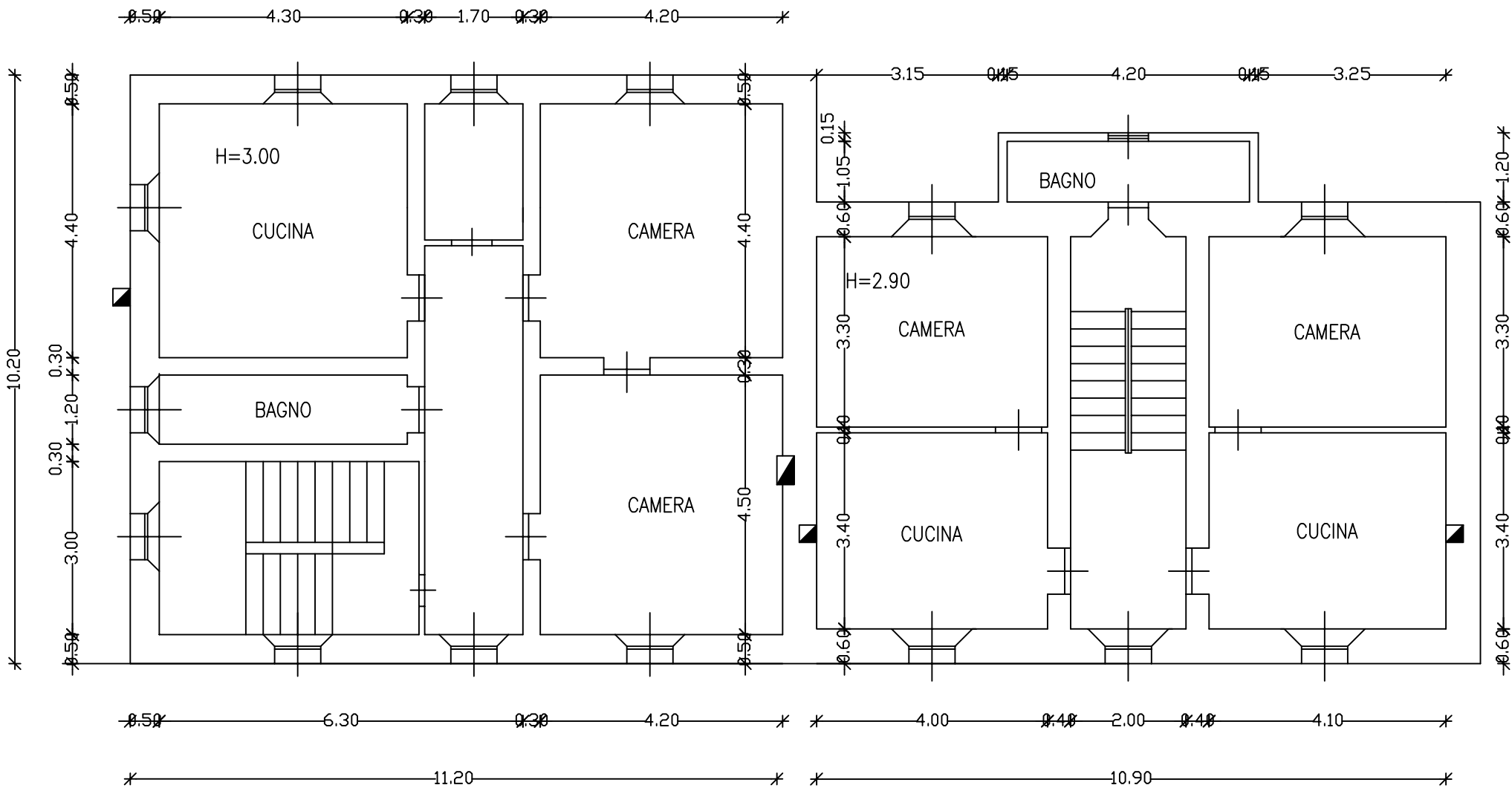
PIANO SECONDO
